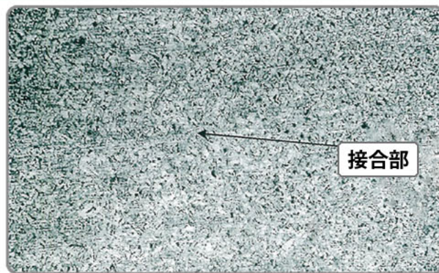
溶接部ミクロ写真 (X400)
