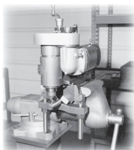
ベンチバイスに取り付け、 小径シャフトのキー溝加工 やギアプーラーなど小型 パーツのフライス加工。
