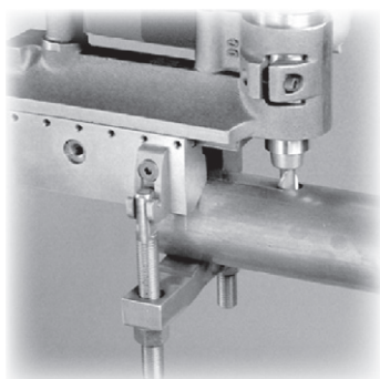
シャフト端への取り付け KM3000の取り付けに必要な シャフト直径は、わずか38.1mm です。
