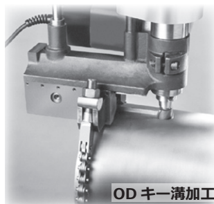
オプションのチェーנקランプ を使用して、最大直径 266mm のシャフトにクランプ。
