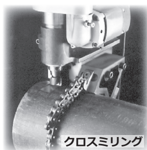
クロスミルアダプター（オ プション）を使用して、ド リルパイプを加工。
