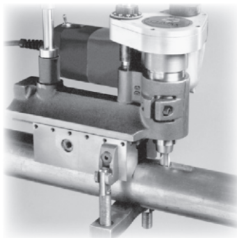
シャフトの中間部分への 取り付け 機械の水平出しを行い、長いキー 溝を加工することができます。
