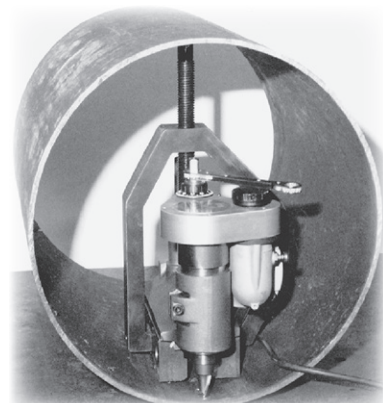
固定治具を用いて、大型タービンな どの内周面をキー溝またはスロット 加工。
