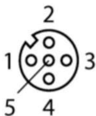
ケーブル側：ピン配置M12,5ピン Aコード,メスコネクタ(ソケット側)
