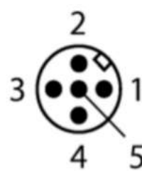
マグネット側：ピン配置M12,5ピン Aコード,オスコネクタ(ピン側)
